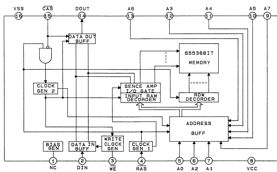
IC303 LM3364K-15
